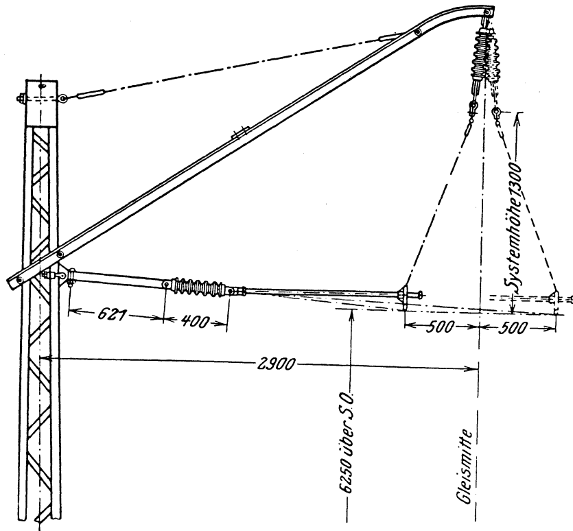
Z 5.3.1./1 Grafing - Rosenheim: Auslegerstützpunkt
