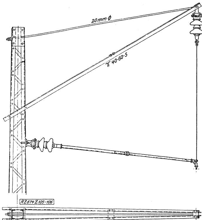
Z 5.2.2./2 BEW-Fahrleitung: Auslegerstützpunkt
