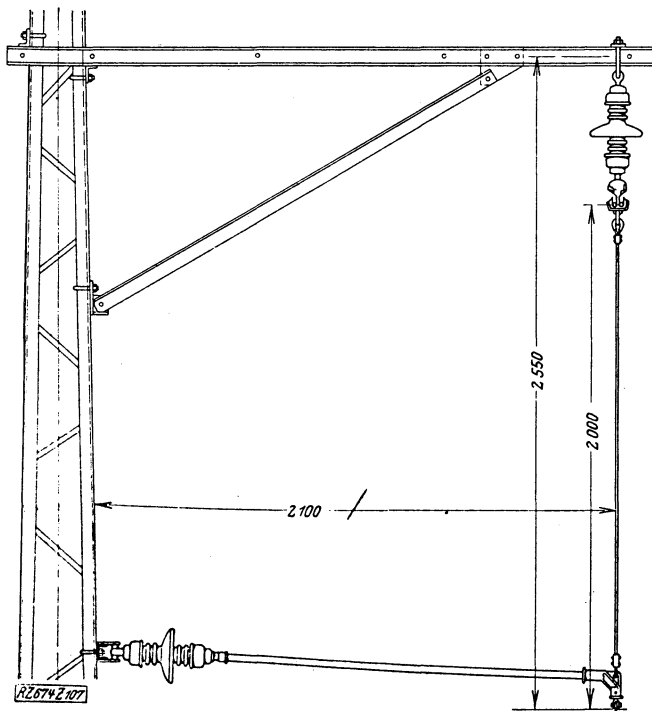
Z 5.2.4.1./2 BBC-Fahrleitung mit lotrechtem Kettenwerk: Auslegerstützpunkt
