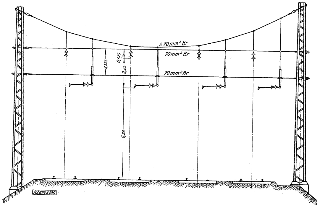
Z 5.2.3./3 SSW-Fahrleitung: Querseilaufhängung
