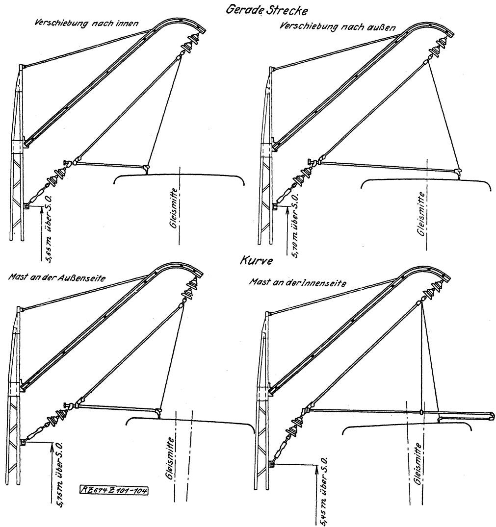
Z 5.2.3./2 SSW-Fahrleitung: Auslegerstützpunkte mit Schrägseilaufhängung
