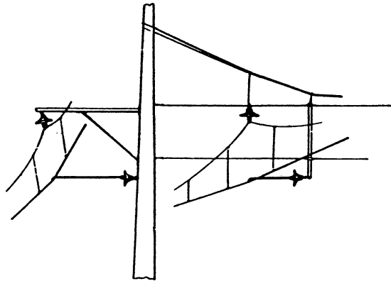
Z 5.2.4.1./1 BBC-Fahrleitung mit lotrechtem Kettenwerk: allgemeine Anordnung
