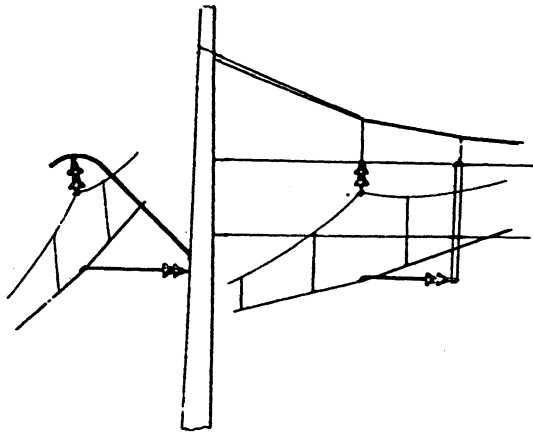
Z 5.2.3./1 SSW-Fahrleitung: allgemeine Anordnung
