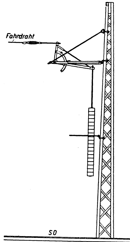
Z 5.3.1./2 Hebelspanner
