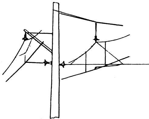
Z 5.2.2./1 BEW-Fahrleitung: allgemeine Anordnung
