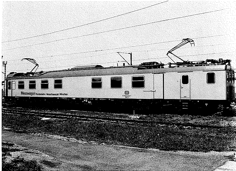
F 1.7./1 Fahrleitungs- meßwagen der DB von 1973 [BZA München]
