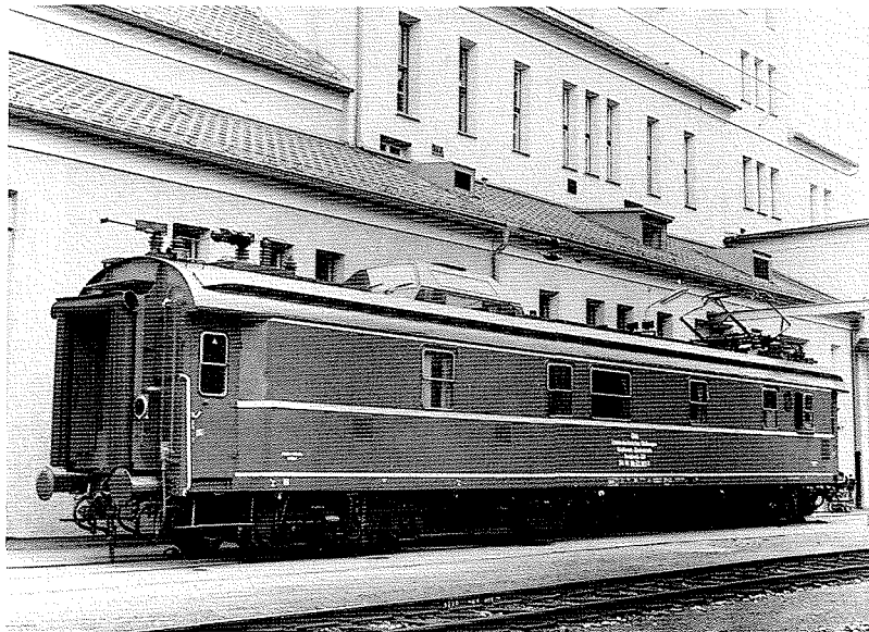
F 1.7./2 Fahrleitungs- meßwagen der ÖBB von 1955 [Petrovitsch]
