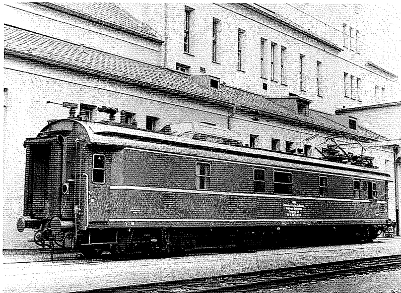
F 1.7./2 Fahrleitungs- meßwagen der ÖBB von 1955 [Petrovitsch]
